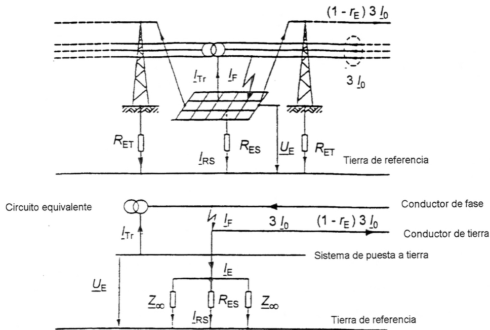
Figura 2. Ejemplo de corrientes de puesta a tierra en una instalación de alta tensión.
